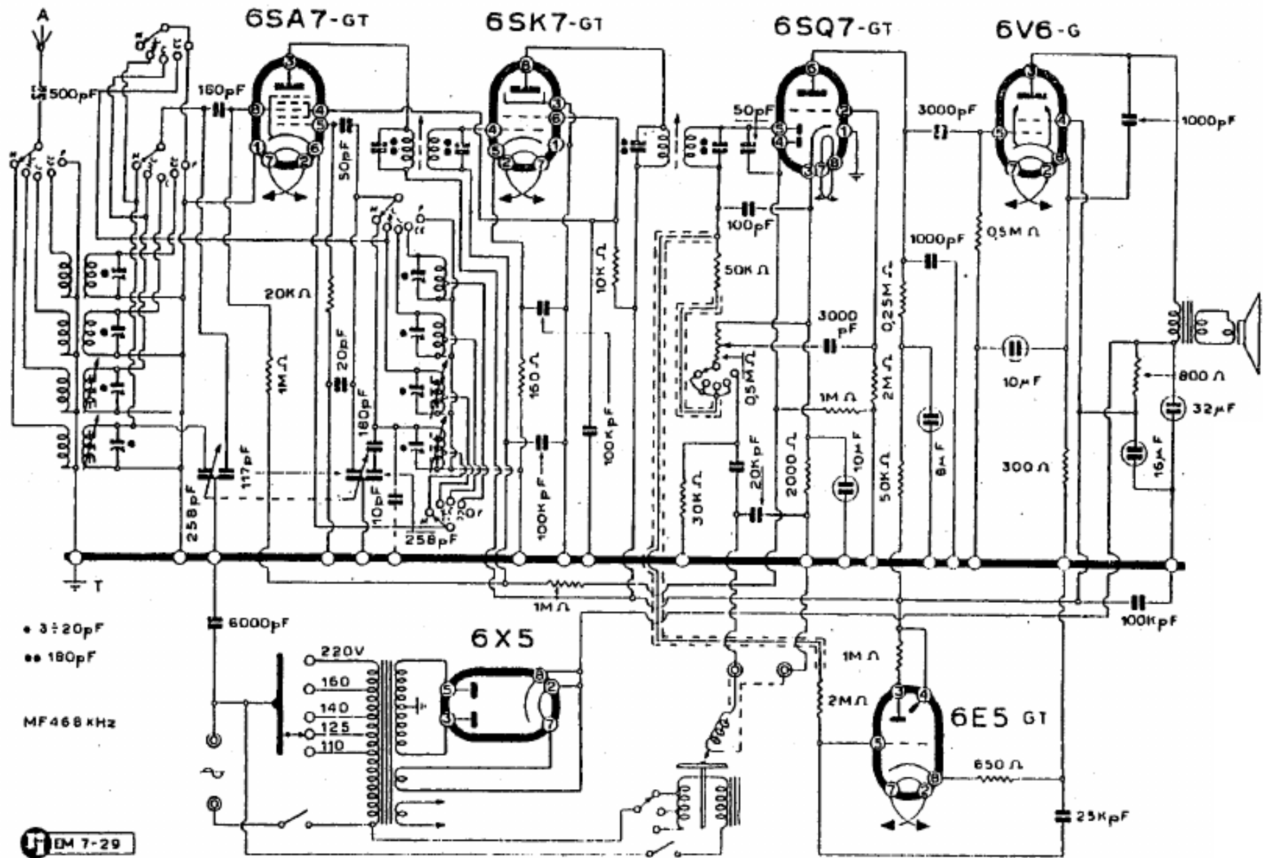
DUCATI ELETTECNICA - Modd. RF 4065 - RF 4965
